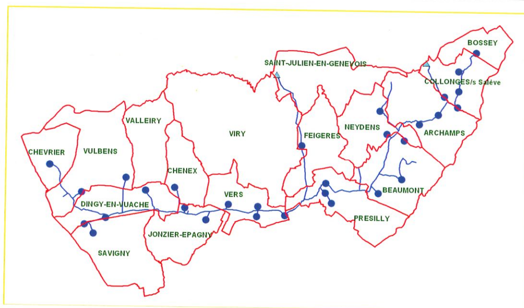
Réseau « primaire » et réservoirs connectés
